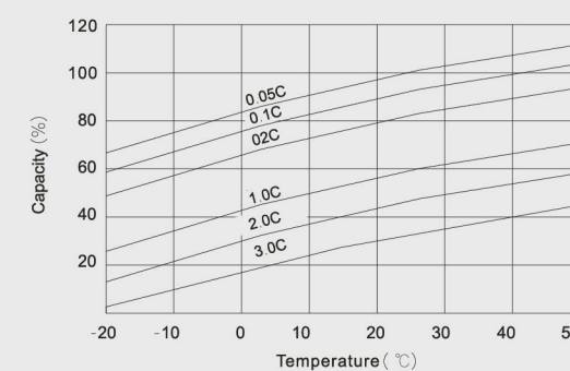
نمودار تأثیر دما بر ظرفیت باتری
